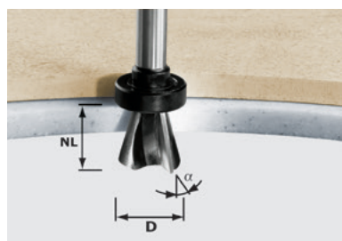
Фреза HW для снятия фаски с верхним опорным подшипником, хвостовик 12 мм HW s = 12
