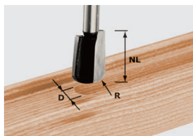
Фреза пазовая U-образная HW, хвостовик 8 мм
