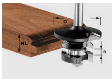
Фреза контрпрофильная гребневая HW, с опорным подшипником, хвостовик 8 мм
