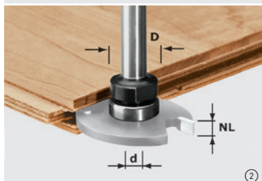
Оснастка для фрезерных шпинделей, хвостик 8 мм
