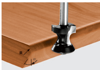
Фрезы скругляющие для снятия фаски HW, с опорным подшипником, хвостовик 8 мм
