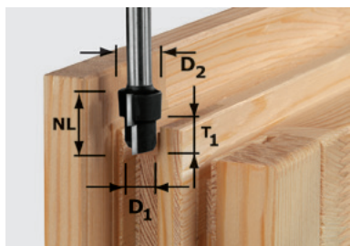
Фрезы для формирования ступенек HW, хвостовик 12 мм
