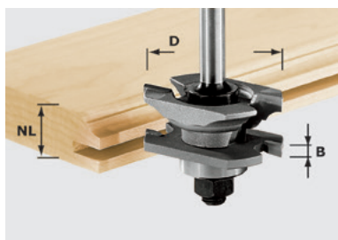
Багетные пазовые фрезы HW с опорным подшипником, хвостовик 8 мм
