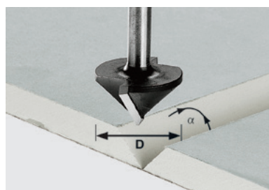
Фрезы по гипсокартону HW, хвостовик 8 мм
