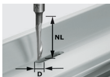
Фреза для обработки алюминиевых сплавов HS, хвостовик 8 мм
