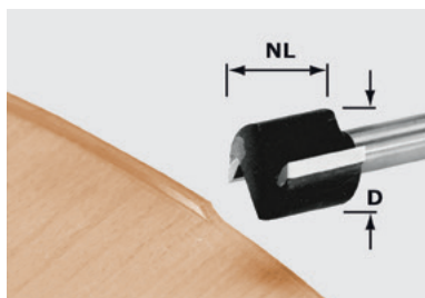
Пригоночная фреза HW, хвостовик 8 мм
