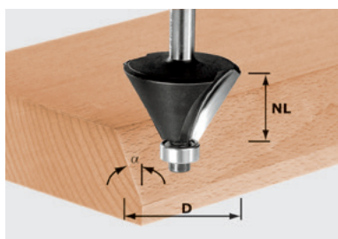
Фрезы для профилирования фасок HW, с опорным подшипником, хвостовик 8 мм
