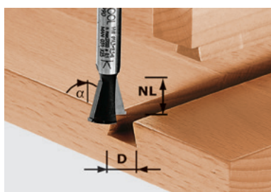
Фрезы «ласточкин хвост» с подрезными ножами, хвостовик 8 мм
