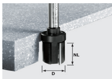
Фрезы пригоночные с верхним подшипником, хвостовик 12 мм HW s = 12
