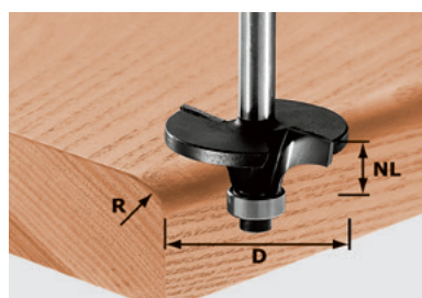
Профильные фрезы HW с опорным подшипником, хвостовик 8 мм
