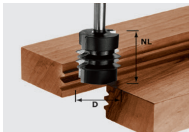
Фреза для сращивания HW, хвостовик 8 мм
