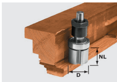
Оконная фреза HW, с неподвижным опорным подшипником сверху
