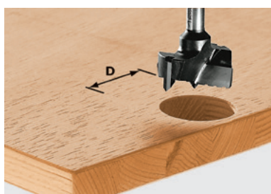
Сверло для гнезд под фурнитуру HW, со стружколомом HW, хвостик 8 мм
