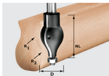
Фрезы для обработки поручней перил HW Profil, хвостовик 12 мм
