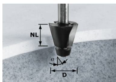
Фрезы для профилирования фасок HW, с опорным подшипником, хвостовик 12 мм HW s = 12
