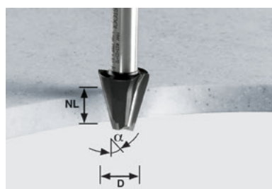
Фрезы HW для профилирования фасок HW s = 12
