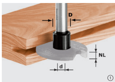
Фрезерные шпиндели для дисковых пазовых фрез HW
