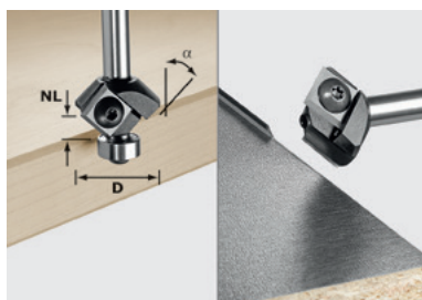
Фреза для снятия фаски со сменными ножами HW, хвостовик 8 мм
