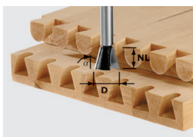
Фрезы конические/ шипрезные фрезы, хвостовик 8 мм
