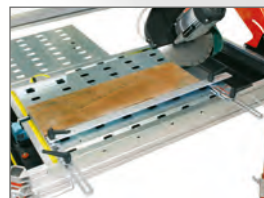
Регулируемая система глубины реза.
