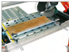
Регулируемая режущая головка
