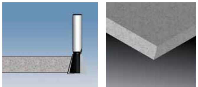
Фреза "ласточкин хвост" 15°
