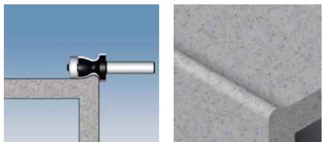
Фреза для формирования кромок с подшипником
