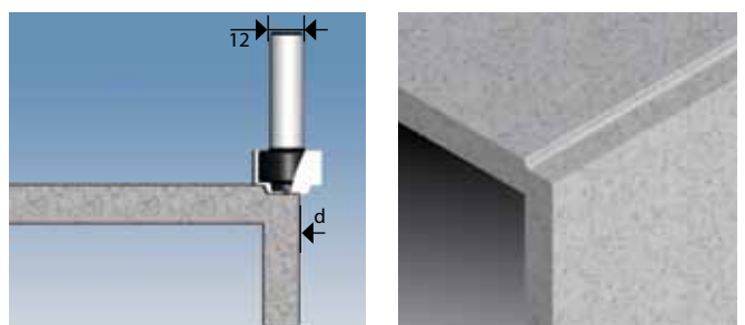
Фреза фасочная для ребер
