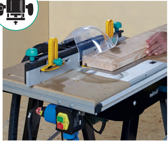
фрезеровочный стол
