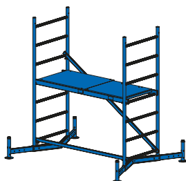
Базовая конструкция № арт. 710116
