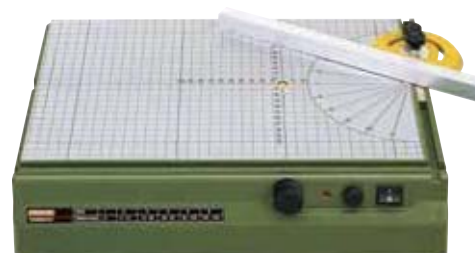
Поворотная направляющая со шкалой и фиксатором. (Немецкий патент 100 00 102.5)
