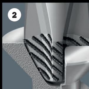
Наконечник Wera Lasertip крепко цепляется за шлиц винта и предотвращает выскальзывание из него
