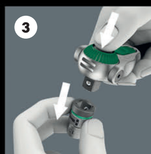
3 Шариковый фиксатор
